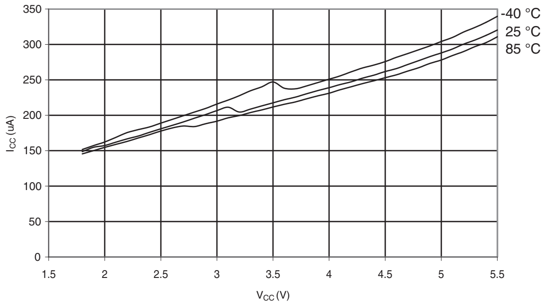
Figure 30-324. ATmega328: ADC Current vs. V CC (AREF = AV CC )
